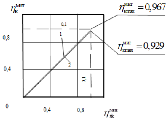
Рис. 1. Графіки залежності для шин: \eta_k^{\text{МИТ}} (\eta_k^{\text{МИТ}}) : 1 – \varphi_{\text{стат}}=0,0325 рад; 2 – \varphi_{\text{стат}}=0,0709 рад
